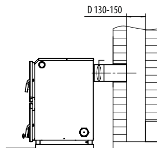
Рис. 10 Присоединение котла к кирпичному дымоходу.
